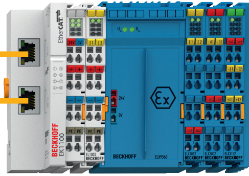
ELX 端子模块: 可以直接连接本质安全型传感器和执行机构
