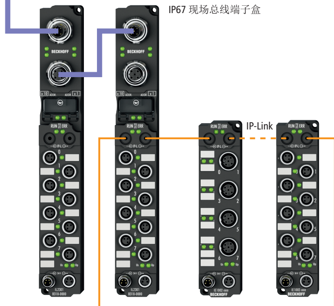
IP67 现场总线端子盒 紧凑型端子盒 耦合器端子盒 扩展端子盒 IP-Link
