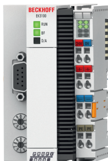
总线耦合器（如 PROFIBUS），适用于 EtherCAT 端子模块
