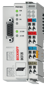
BK 系列总线耦合器，用于连接总线端子模块和现场总线
