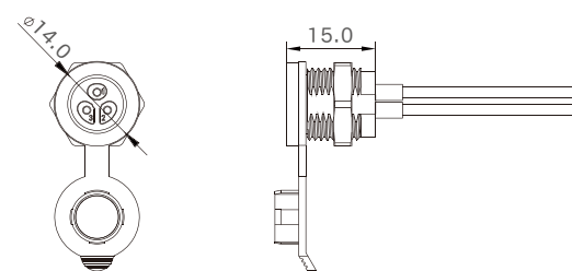
母端图
