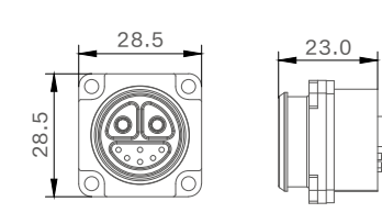
母端图
