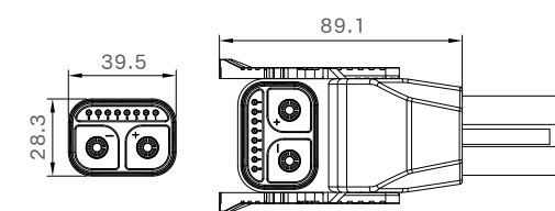
公端图
