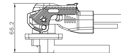
互配图
