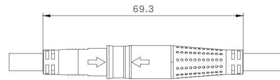
互配图
