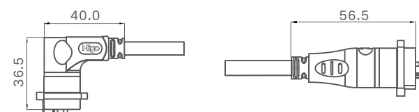
互配图
