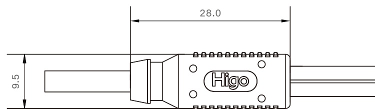
产品尺寸
