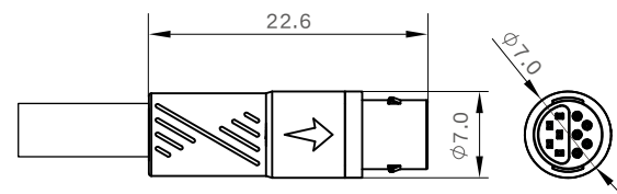
母端图
