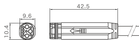
母端图
