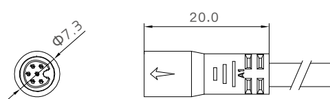
母端图
