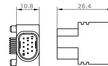
公端图
