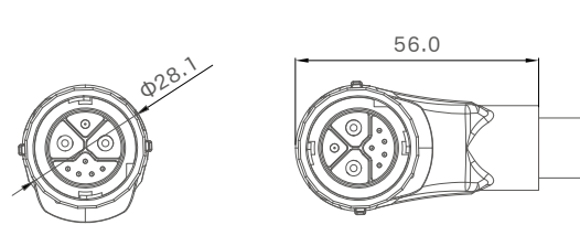
公端图
