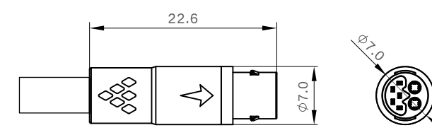
母端图
