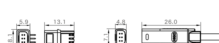
公端图
