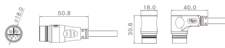
公端图
