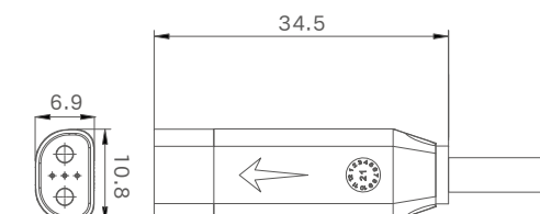
公端图
