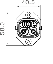
母端图
