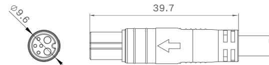
公端图
