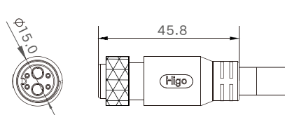
母端图
