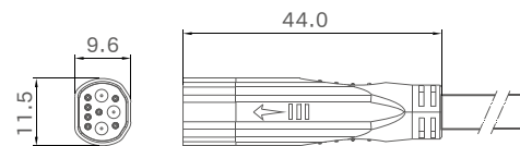
公端图
