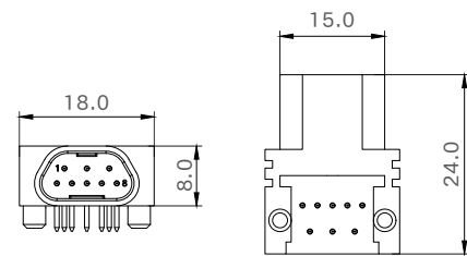
公端图
