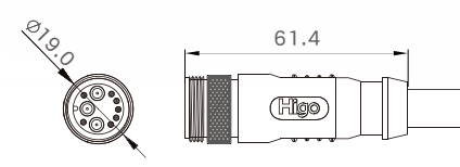
公端图
