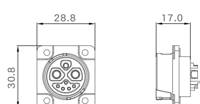
母端图
