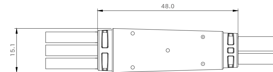
产品尺寸
