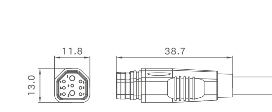
母端图
