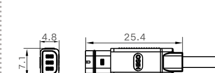
母端图
