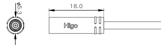
公端图
