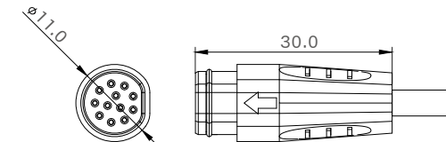
母端图
