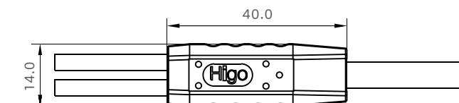
产品尺寸
