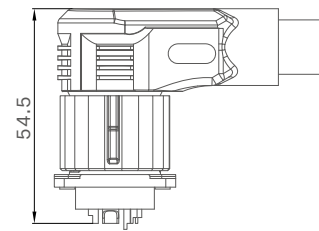
互配图
