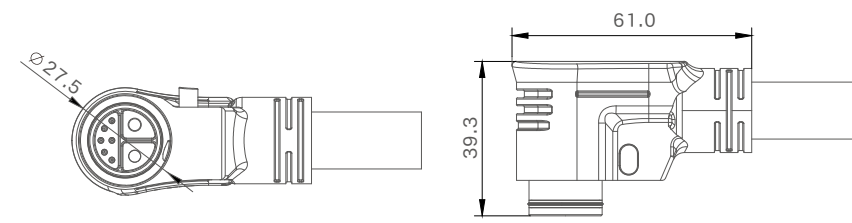
公端图
