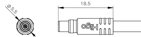
母端图
