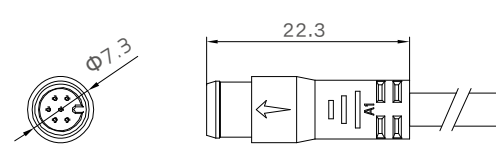
公端图
