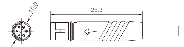
母端图
