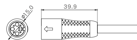
母端图
