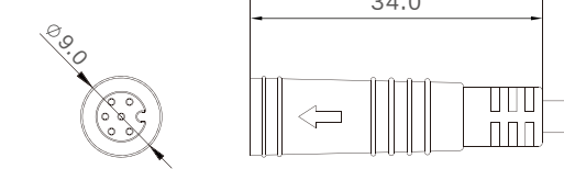
母端图
