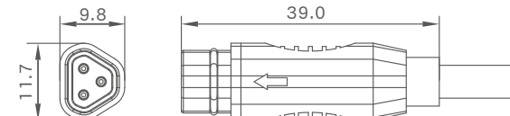
公端图
