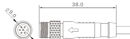
公端图
