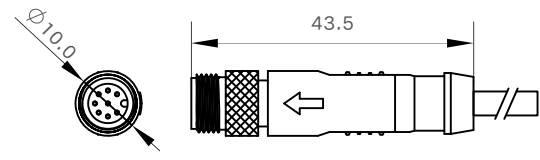
公端图
