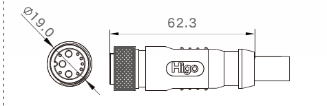
母端图
