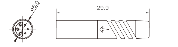
公端图
