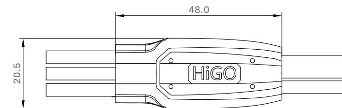
产品尺寸
