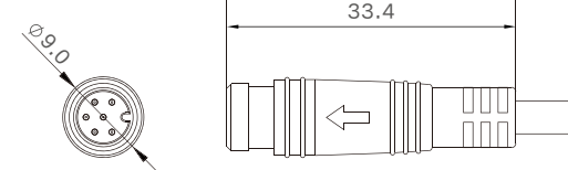
公端图
