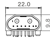
母端图
