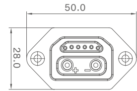
母端图
