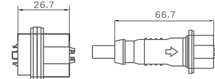
互配图
