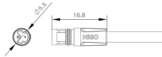
母端图
