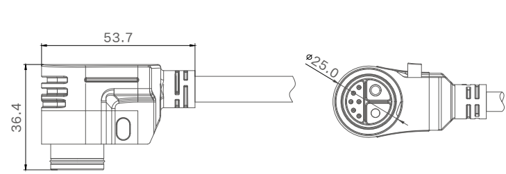
公端图
