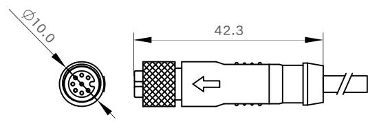
母端图
