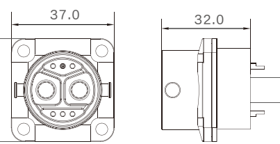
母端图
