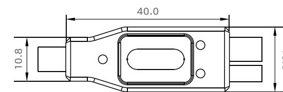
产品尺寸
