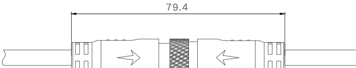
互配图
