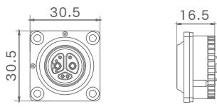
母端图
