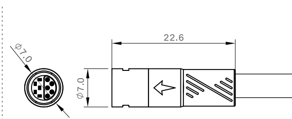
公端图
