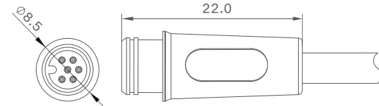
公端图
