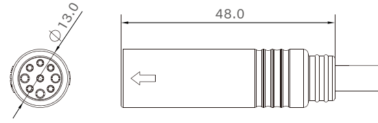
母端图
