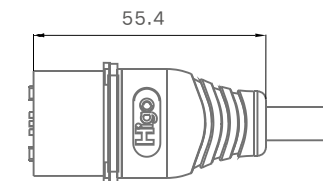
互配图
