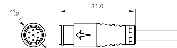
公端图
