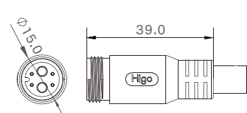
公端图
