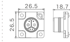
公端图
