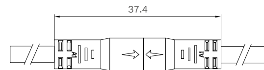
互配图
