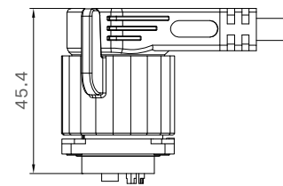
互配图
