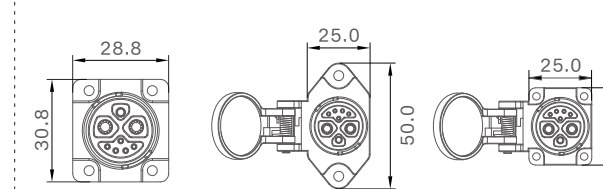
母端图
