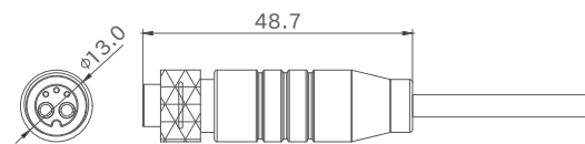
母端图
