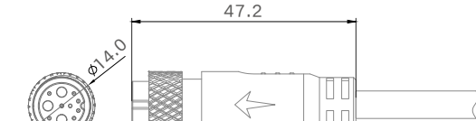
母端图
