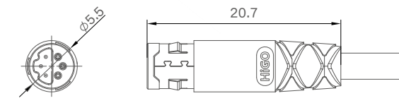
母端图
