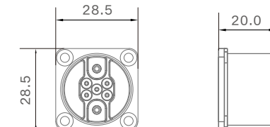
公端图
