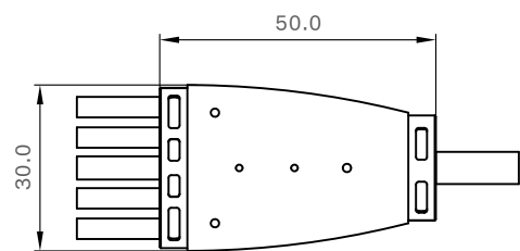
产品尺寸
