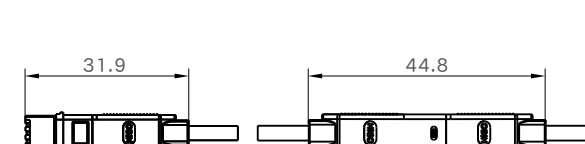
互配图
