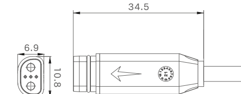
母端图
