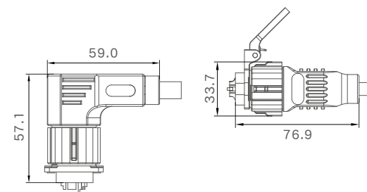
互配图
