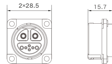
母端图
