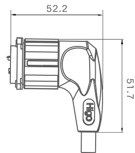
互配图
