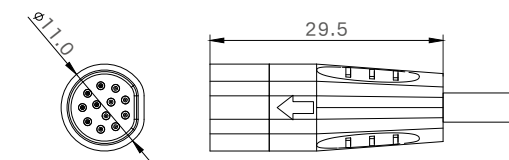
公端图
