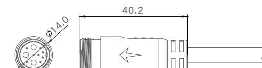
公端图
