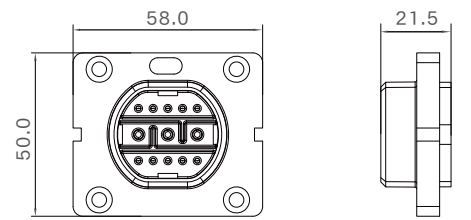
母端图
