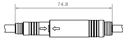
互配图
