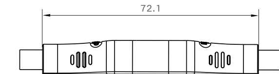
互配图
