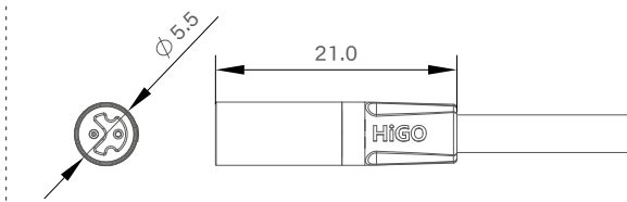
公端图
