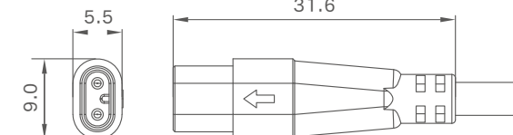
公端图
