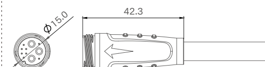
公端图
