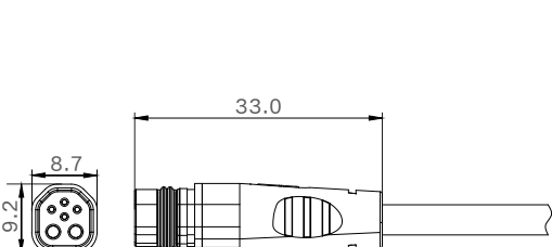
母端图
