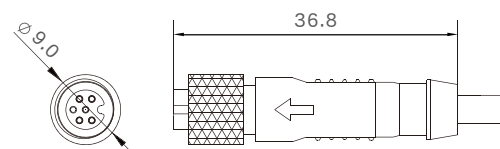
母端图
