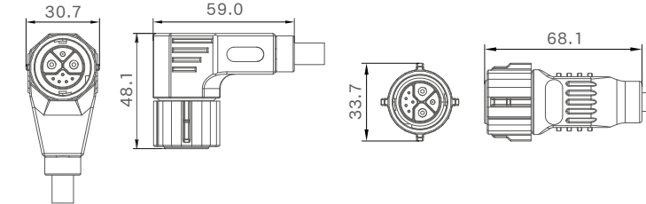
公端图
