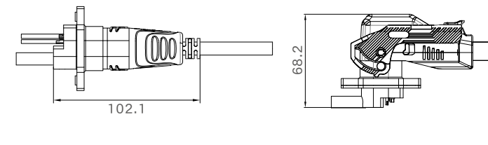
互配图
