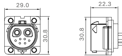
母端图
