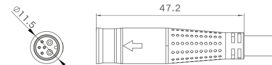
母端图
