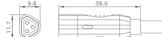
母端图
