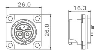
母端图
