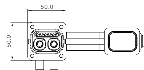
母端图
