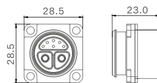
母端图
