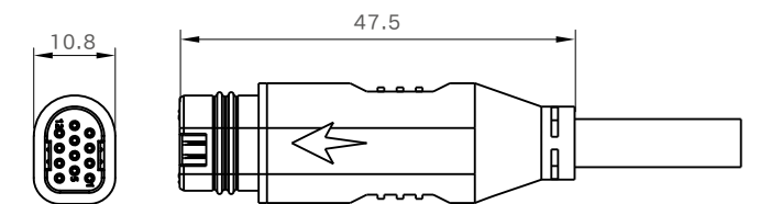
母端图
