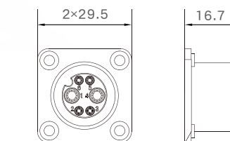
母端图
