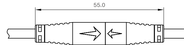
互配图
