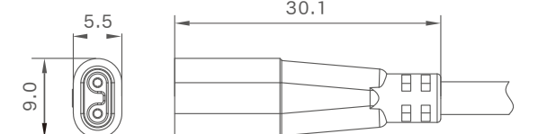
母端图
