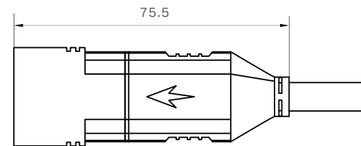
互配图
