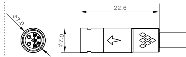
公端图
