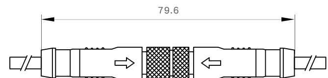
互配图
