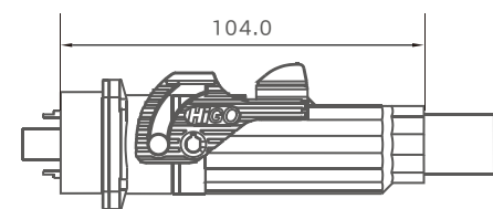
互配图
