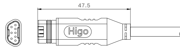
母端图
