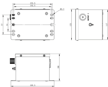
QP-HD-I/QP-HD-II/QP-HK电源尺寸
