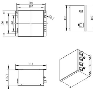
QP-HD-IV电源尺寸
